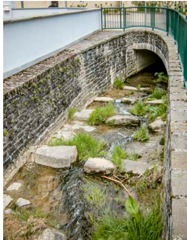
Aufwertung der Gewässersohle des Burbichs in Arsdorf durch bewachsene Kiesbänke (links) und Störsteine (rechts). (Fotos: Planungsbüro Zumbroich, 2019)
